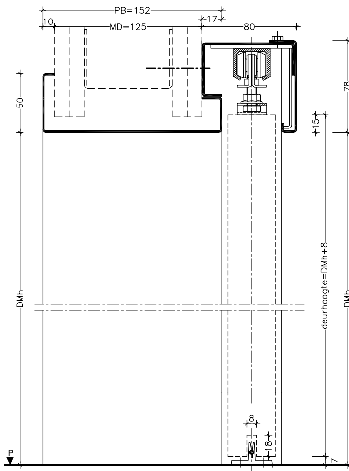
Doorsnede 3-4
