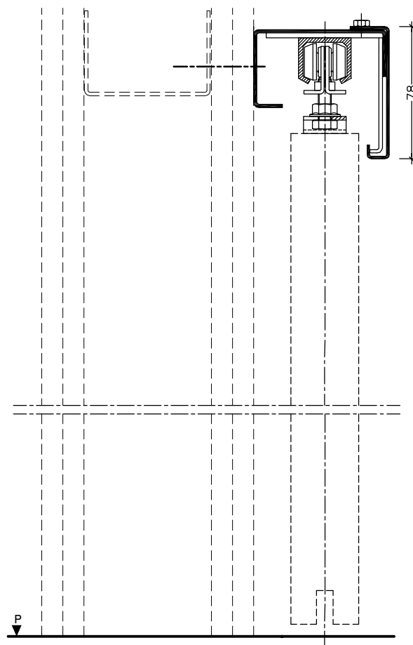
Doorsnede 5-6
